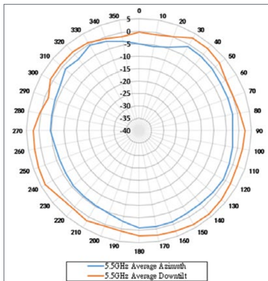
Plano acimutal (vista superior) - BLE
