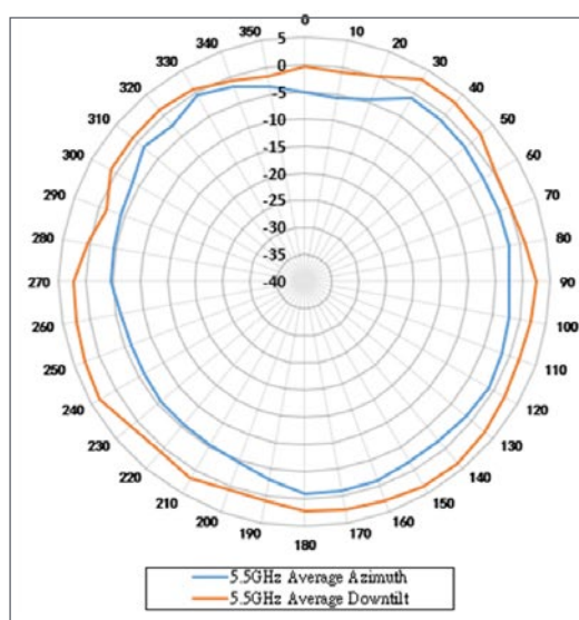
Plano acimutal (vista superior) - 5 GHz
