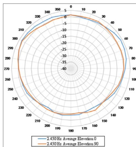
Plano de elevación (vista lateral) - 2,4 GHz
