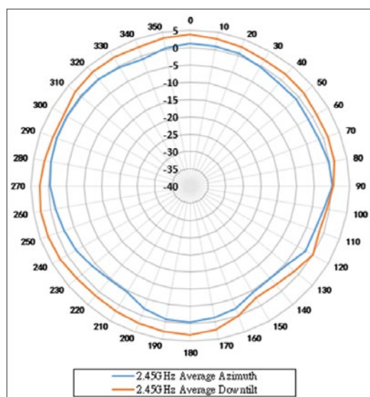
Plano acimutal (vista superior) - 2,4 GHz
