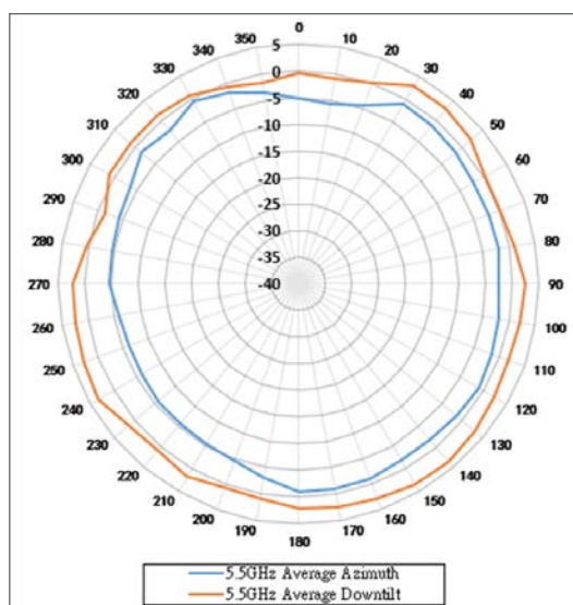
Plano acimutal (vista superior) - 6 GHz
